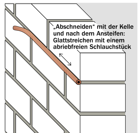
Bild 3/17: Fugenglattstrich
