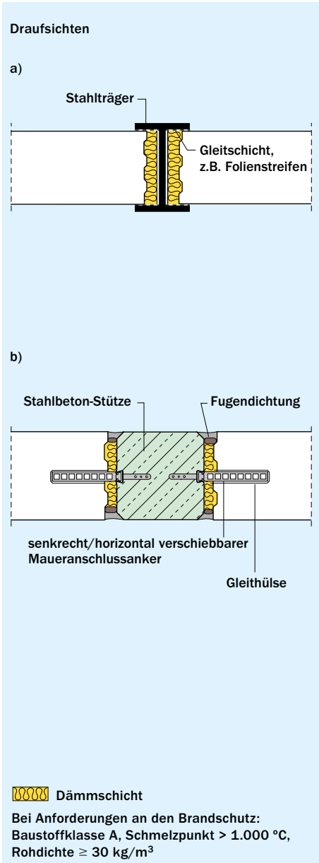
Bild 35 Anschluss an Zwischenstütze (Aussteifungsstütze)
