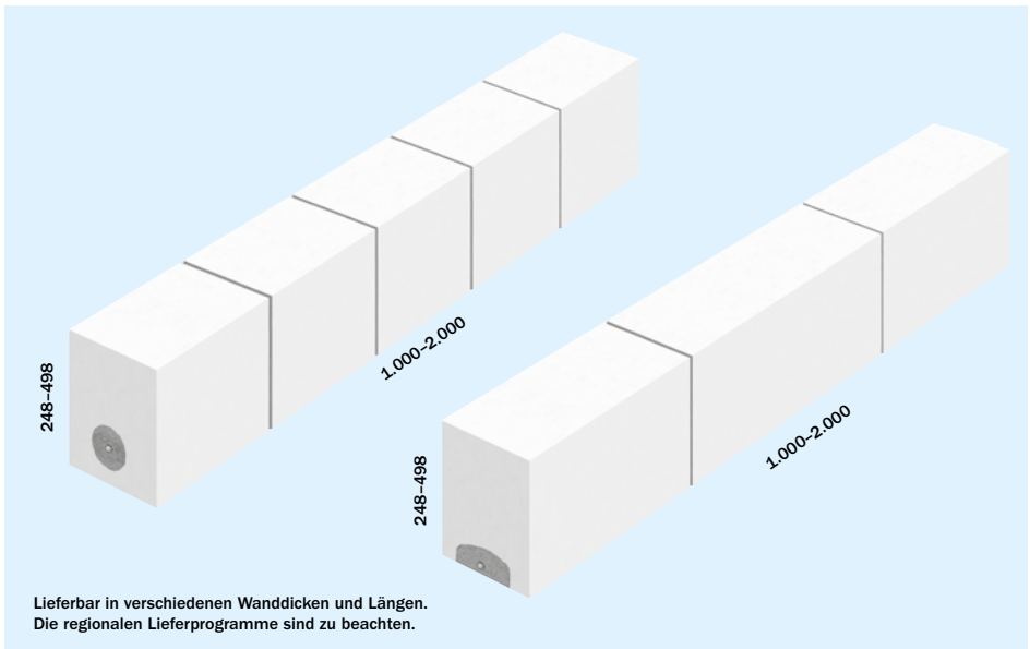
Bild 13 KS-Fertigteilstürze nach allgemeiner bauaufsichtlicher Zulassung (abZ)
