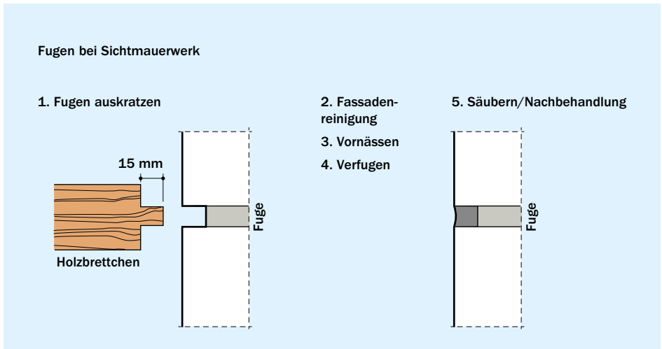
Bild 30 Vor dem Erhärten des Mauermörtels werden die Fugen mindestens 15 mm tief ausgekratzt und später mit Fugenmörtel ausgefügt. Die Steinbreite muss dabei \geq 105 mm sein.
