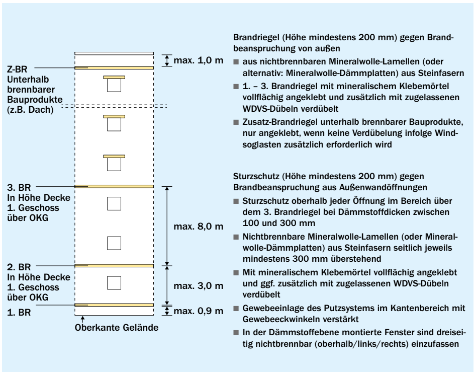
Bild 18 Schwerentflammare WDVS mit EPS ( d \leq 300 mm) – Ausbildung mit umlaufenden Brandriegeln sowie Schutz der Fensteröffnungen
