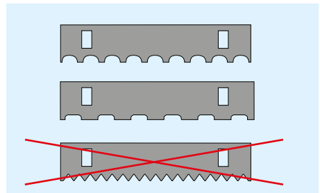
Bild 3 Beispiele verschiedener Zahnschienen für Dünnbettmörtel
