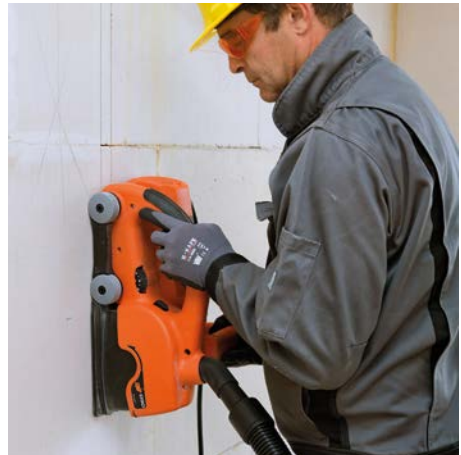
Bild 3 Vertikales Fräsen
